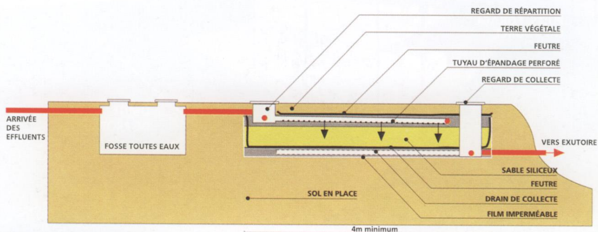
COUPE LONGITUDINALE
